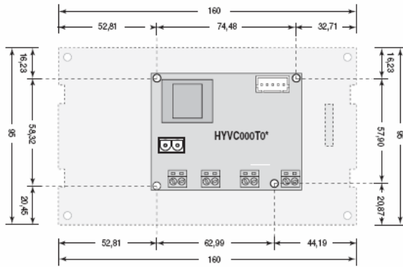
główne wymiary płytki elektronicznej
